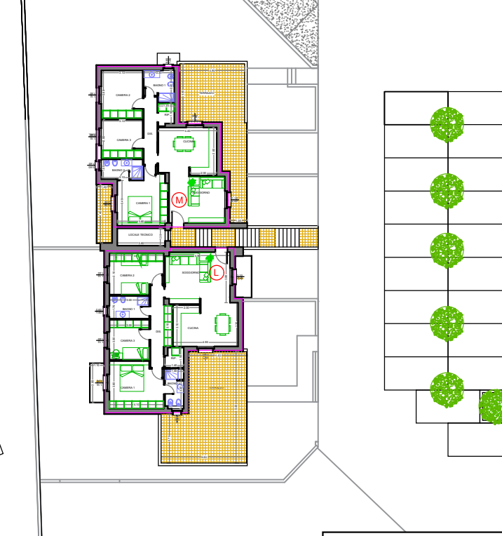
PIANO PRIMO - SCALA 1:200
